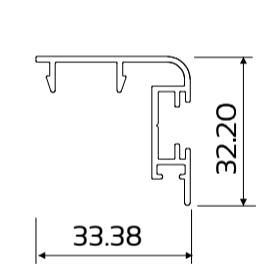
DIE No. W72204 Clip-On Interlocker
