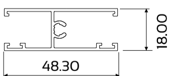
DIE No. W72248 Sash Frame Transom
